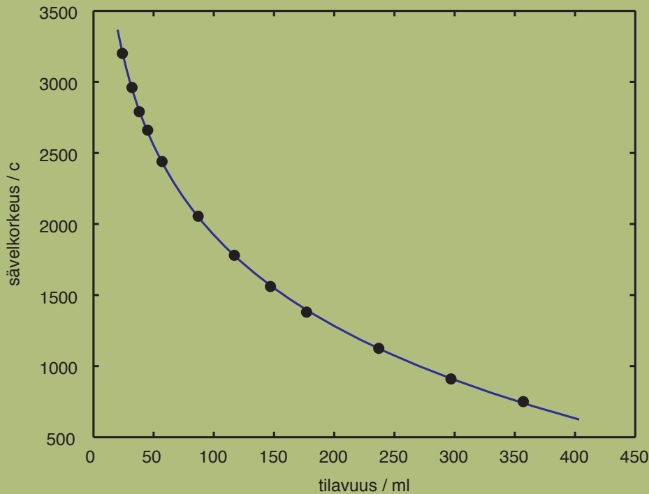
Kuva 1: Mitattu sävelkorkeus pullossa olevan ilmamäärän tilavuuden funktiona.
