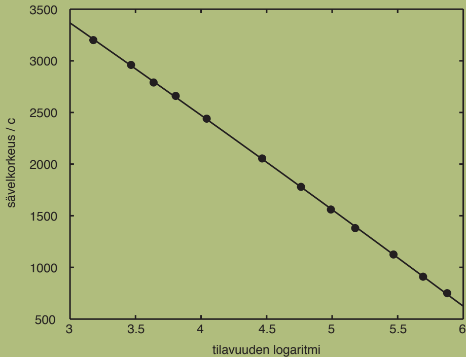
Kuva 2: Mitattu sävelkorkeus pullossa olevan ilmamäärän tilavuuden logaritmin funktiona.
