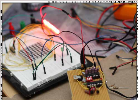
Ohjauselektronikan testaamista
